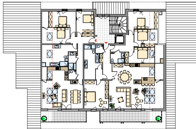
2e verdieping (penthouses)
